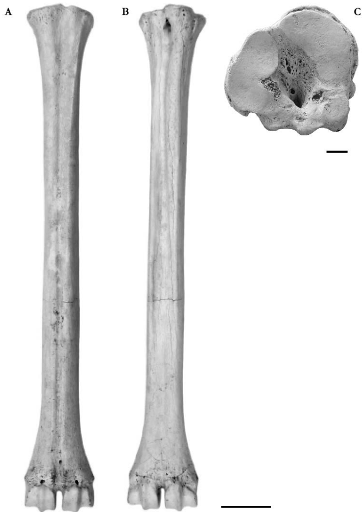
Figura 3. Mt III-IV izquierdo de Mitilanotherium sp. (FP1-2002-1108). A: vista dorsal; B: vista plantar; C: vista proximal. Escala gráfica en A y B: 5 cm. Escala gráfica en C: 1 cm.
