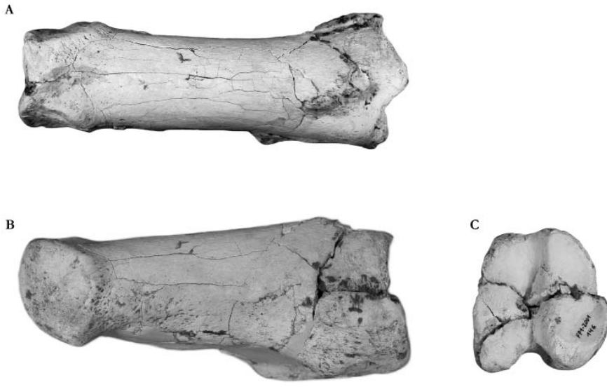
Figura 2. Falange primera anterior de Mitilanotherium sp. (FP1-2001-0146). A: vista dorsal; B: vista medial; C: vista proximal. Escala gráfica: 1 cm.
