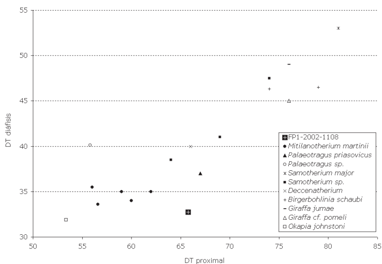
Figura 6. Representación bivariante del diámetro transversal (DT) de la epífisis proximal frente al diámetro transversal de la diáfisis en el Mt III-IV de distintos jiráfidos fósiles y actuales. Datos tomados de tabla 1, Crusafont (1952), Bolomey (1965), Samson y Radulesco (1966), Geraads (1981), Godina y Baygusheva (1985), Geraads (1994), Athanassiou (1996), Kostopoulos (1996), Geraads (1998) y Geraads y Güleç (1999). Se incluyen además las dimensiones del ejemplar de Okapia johnstoni cedido temporalmente por el Muséé Royal de l'Afrique Centrale de Tervuren (Bélgica).
