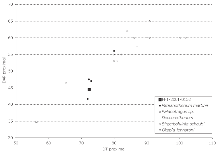
Figura 5. Representación bivariente del diámetro transversal (DT) frente al diámetro antero-posterior (DAP) de la epífisis proximal del Mc III-IV en distintos jiráfidos fósiles y actuales. Datos tomados de tabla 1, Crusafont (1952), Bolomey (1965), Samson y Radulesco (1966) y Kostopoulos (1996). Se incluyen además las dimensiones del ejemplar de Okapia johnstoni cedido temporalmente por el Muséé Royal de l'Afrique Centrale de Tervuren (Bélgica).
