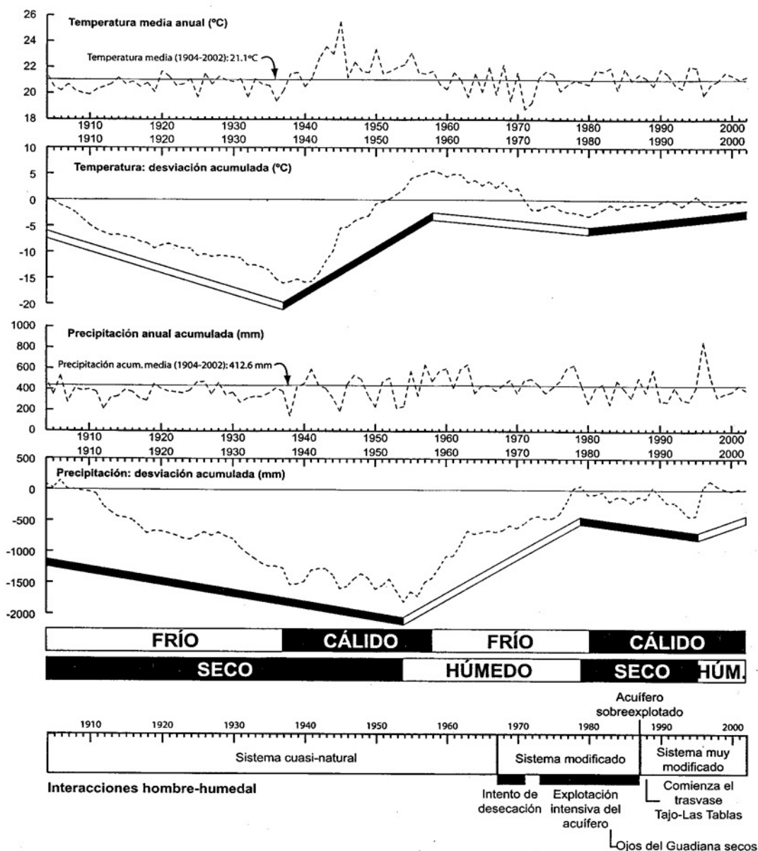
FIGURA 3. Evolución temporal de los valores anuales (precipitación y temperatura) para 1904-2002 y principales acciones del hombre sobre el medio.
